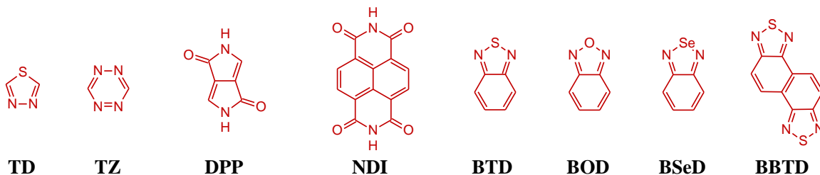
Rysunek 1. Struktury jednostek elektronodonorowych (D) i elektronoakceptorowych (A) półprzewodników organicznych opisanych w rozprawie habilitacyjnej.
