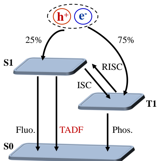
Schemat 1. Schemat idealny przebiegu procesu TADF w urządzeniu OLED. S_0 – stan podstawowy, S_1 – najniższy singletowy stan wzbudzony, T_1 – najniższy trypletowy stan wzbudzony, Fluo. – fluorescencja natychmiastowa, TADF – aktywowana termicznie opóźniona fluorescencja, Phos. – fosforescencja, ISC – przejście międzysystemowe, RISC – odwrotne przejście międzysystemowe.
