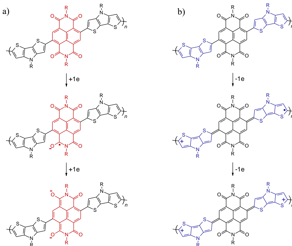
Rysunek 6. Dwuetapowe, dwuelektronowe procesy (a) redukcji i (b) utleniania poli[NDI-(DTP) 2 ].
